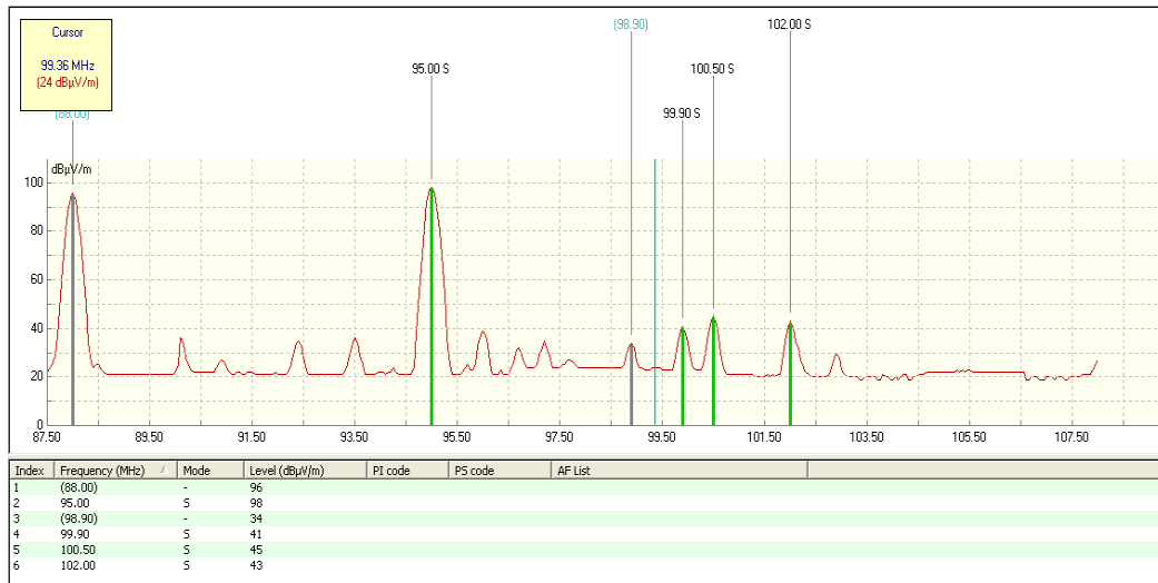
Mynd 5: Mælingar með 5 W afl sendis.
