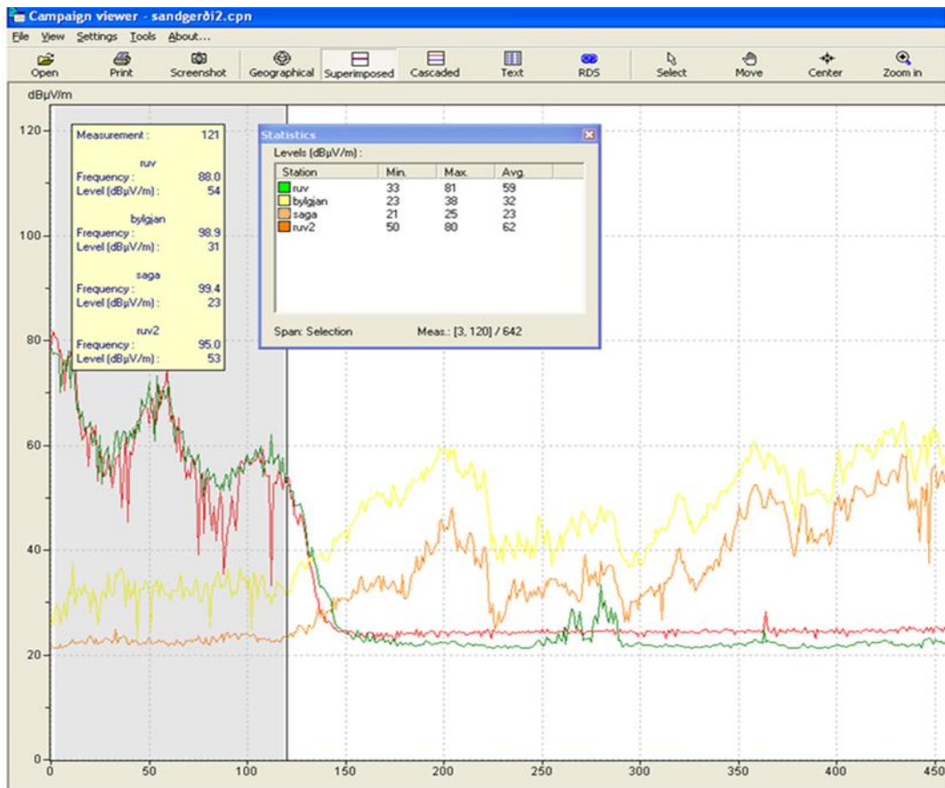
Mynd 6: Meðaltalsmælingar innan Sandgerðisbæjar
