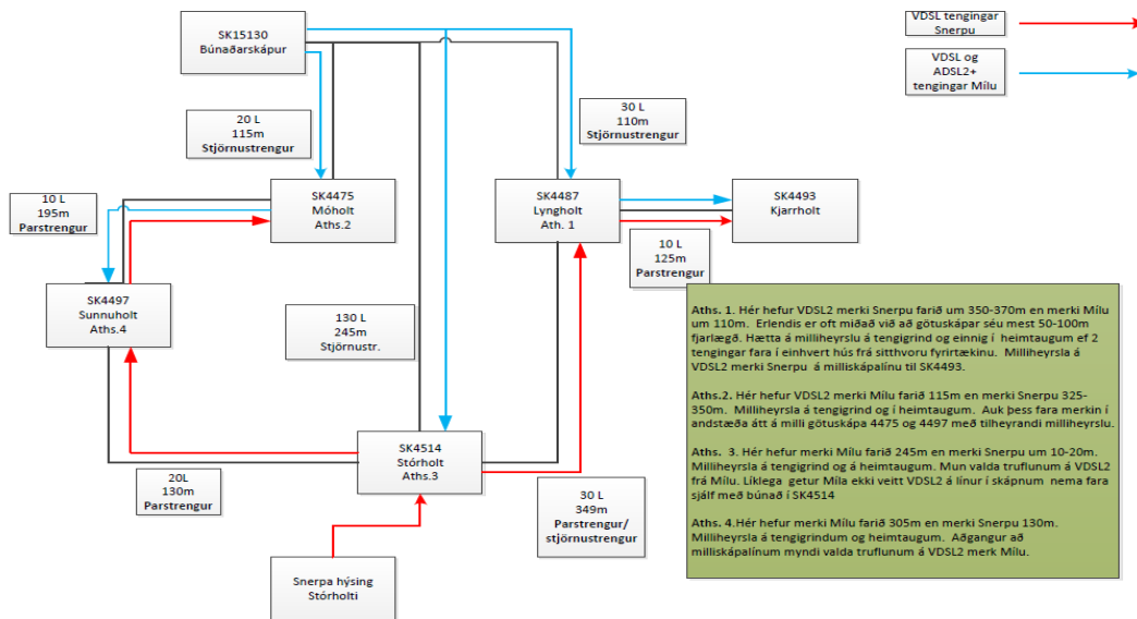
Mynd sem sýnir þann hluta götuskápkakerfis Milu sem deilan snýst um í Holtahverfi á Ísafirði eftir að Míla setur upp búnað í götuskaða á svæðinu.
