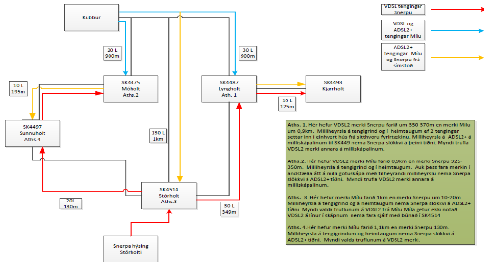
Mynd sem sýnir þann hluta götuskápkakerfis Milu sem deilan snýst um í Holtahverfi á Ísafirði áður en Míla setur upp búnað í götuskaða á svæðinu.
