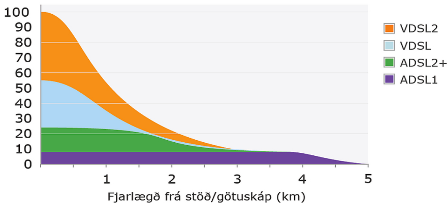
Fræðileg hámarksafköst á xDSL samböndum mv. vegalengd.
